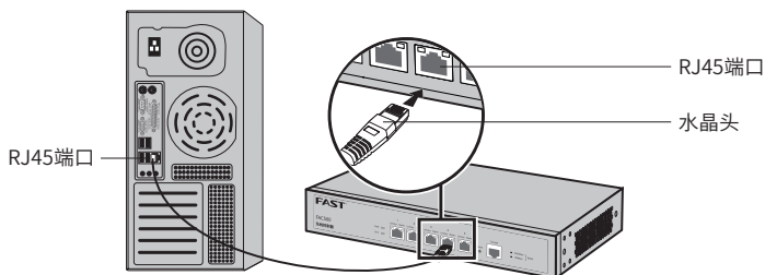
图4-1 无线控制器连接线缆示意图
